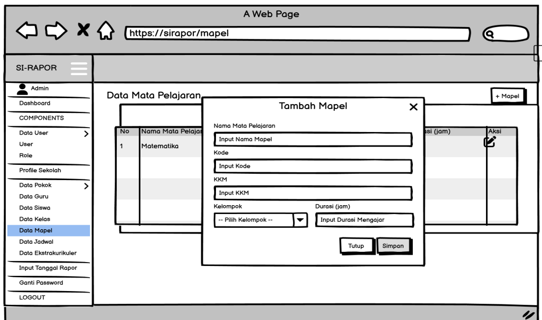
Gambar 1.58 Tampilan modal form tambah data mapel
