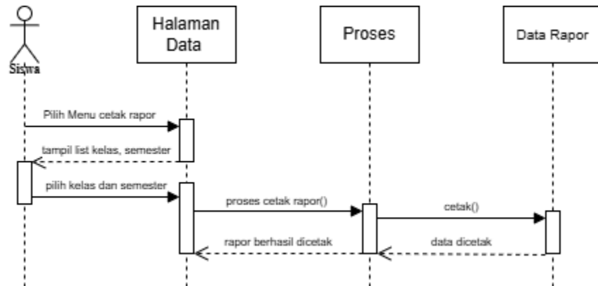
Gambar 1.33 Sequence diagram siswa cetak rapor
