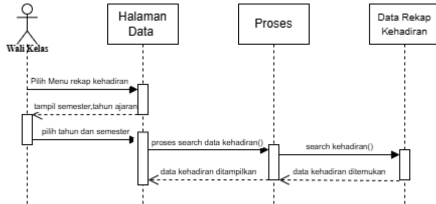
Gambar 1.30 Sequence diagram wali kelas kelola data kehadiran siswa
