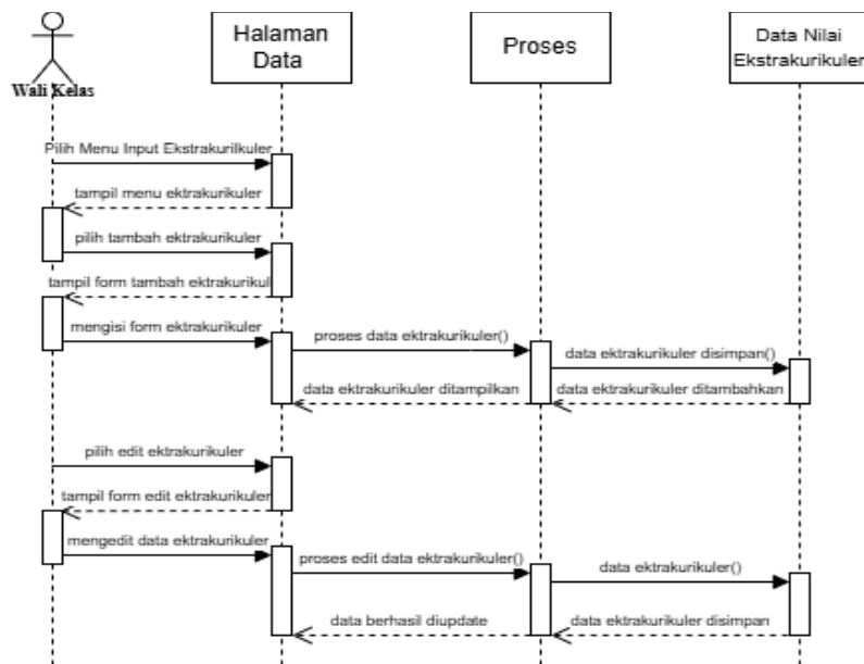
Gambar 1.29 Sequence diagram wali kelas kelola data ekstrakurikuler siswa
