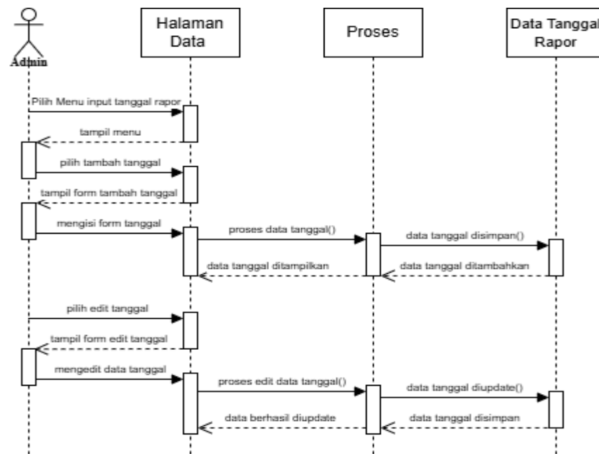
Gambar 1.23 Sequence diagram admin kelola data tanggal rapor
