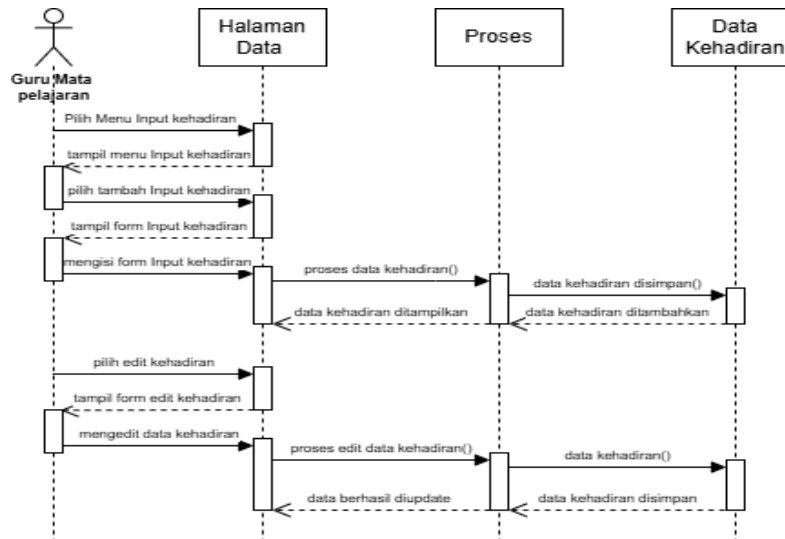
Gambar 1.24 Sequence diagram guru mata pelajaran kelola data kehadiran siswa
