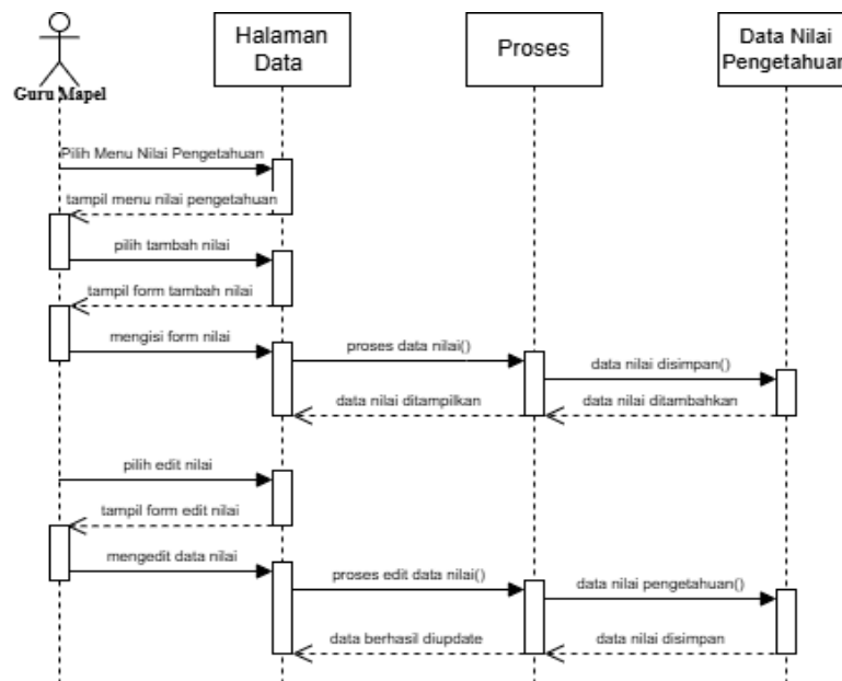
Gambar 1.25 Sequence diagram guru mata pelajaran kelola data nilai pengetahuan siswa
