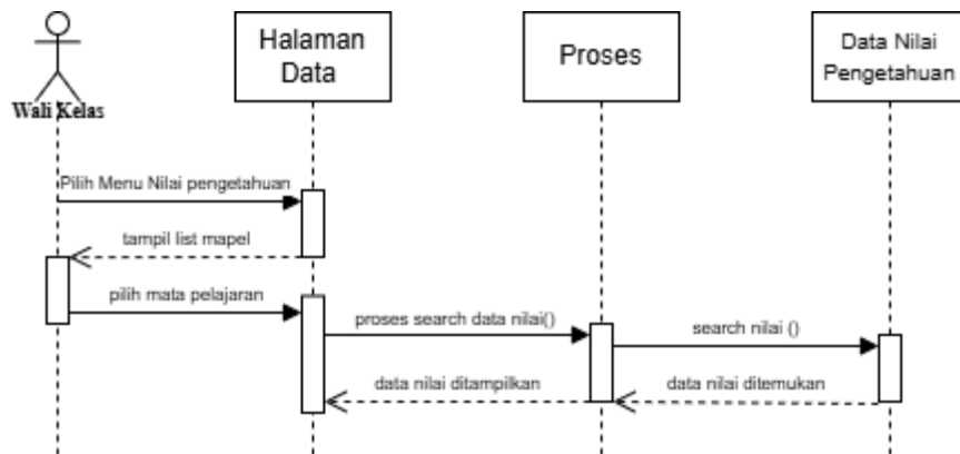
Gambar 1.27 Sequence diagram wali kelas kelola data nilai pengetahua siswa
