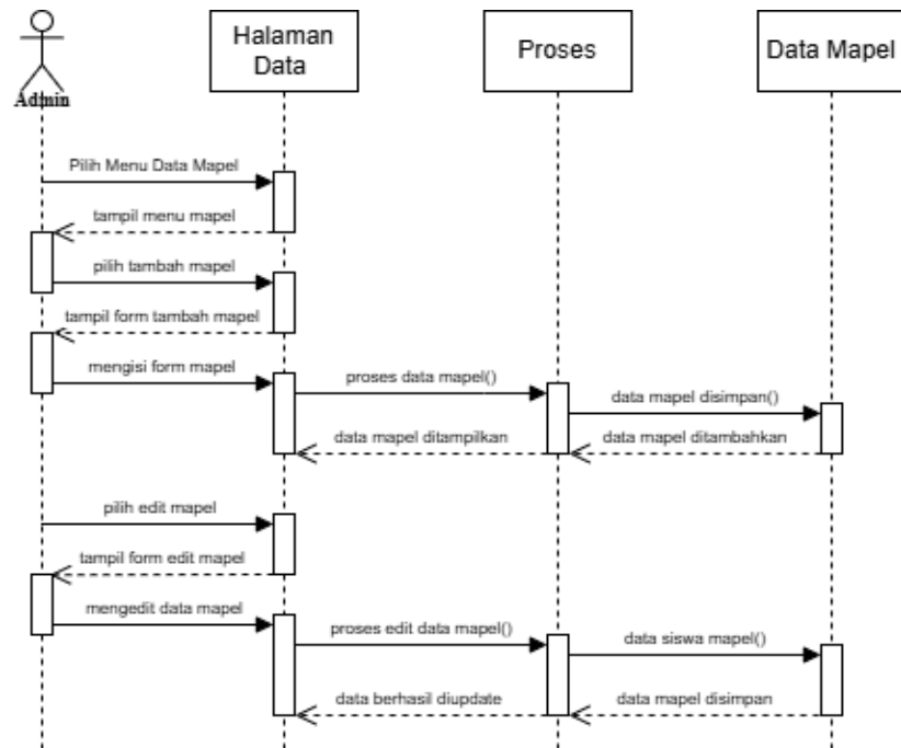
Gambar 1.20 Sequence diagram admin kelola data mata pelajaran
