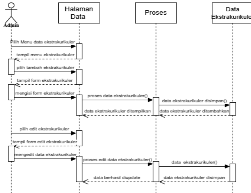
Gambar 1.22 Sequence diagram admin kelola data ekstrakurikuler
