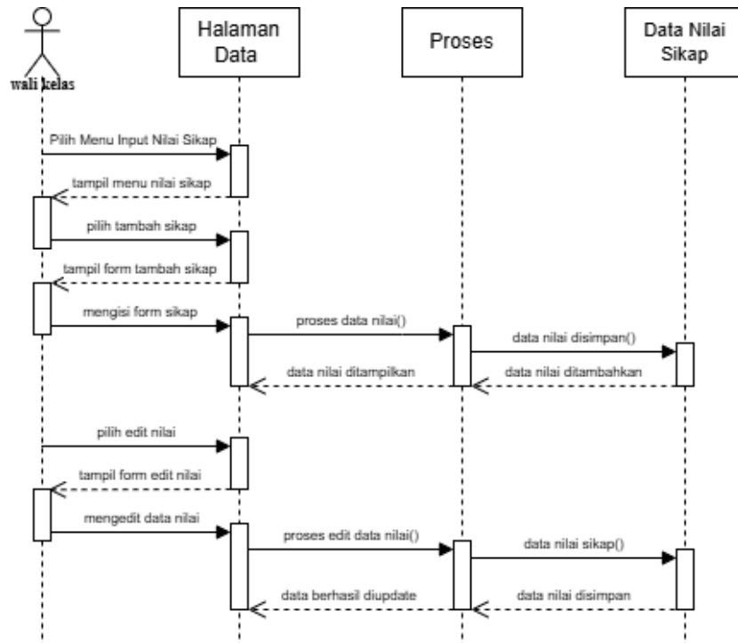
Gambar 1.26 Sequence diagram wali kelas kelola data nilai sikap siswa
