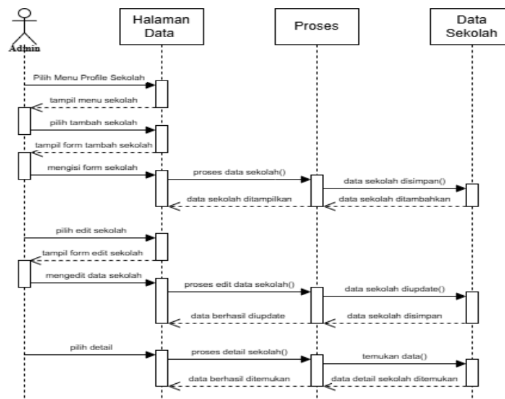
Gambar 1.16 Sequence Diagram Admin Kelola Data Sekolah
