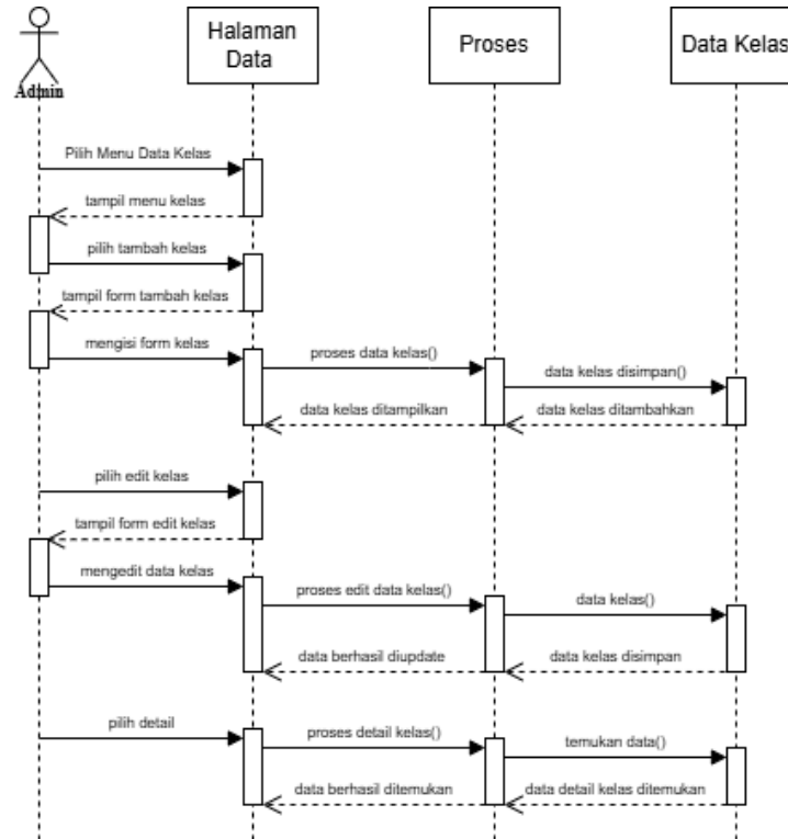
Gambar 1.19 Sequence diagram admin kelola data kelas
