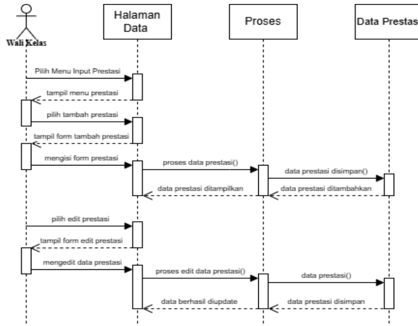
Gambar 1.28 Sequence diagram wali kelas kelola data prestasi siswa
