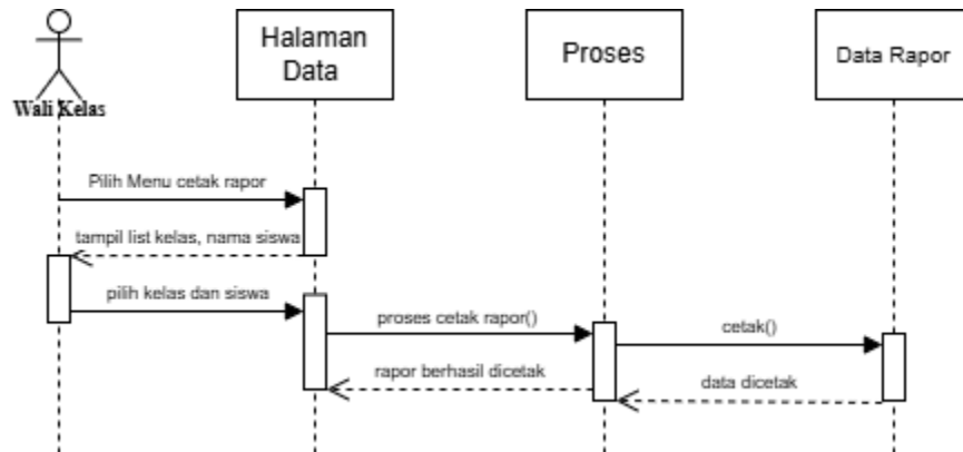
Gambar 1.31 Sequence diagram wali kelas cetak rapor siswa
