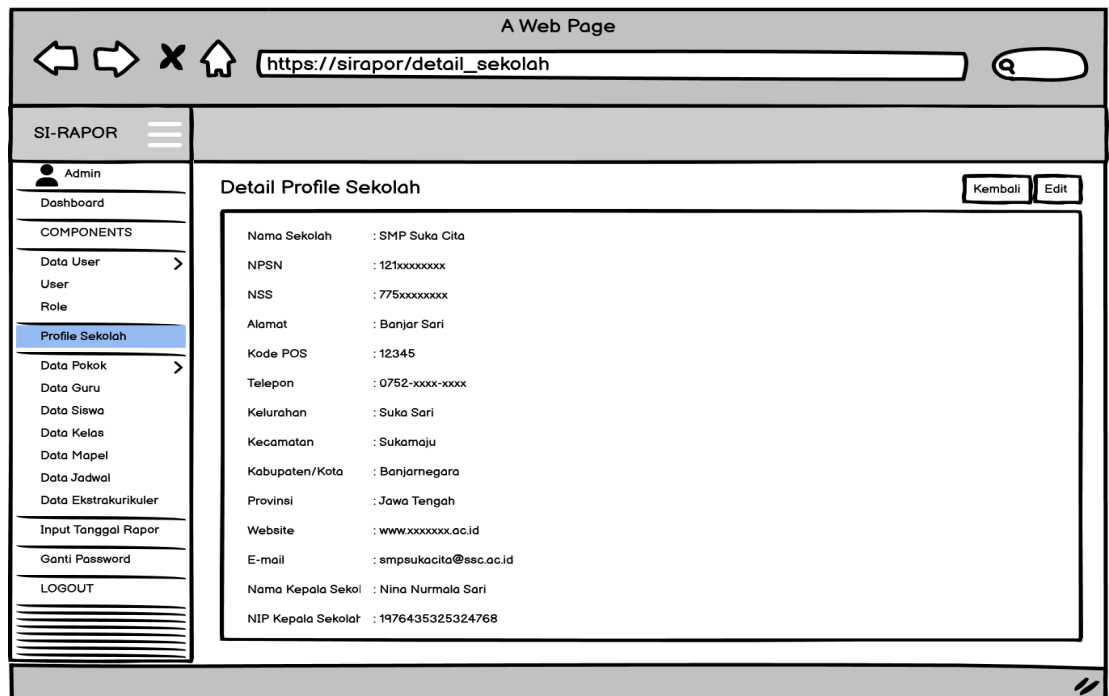
Gambar 1.44 Tampilan detail profile sekolah
